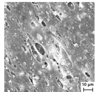
Même vue microscopique d'un écran de sous-toiture conventionnel. Le procédé de production consiste à étirer le film de PP et à y ajouter du carbonate de calcium. Cela crée des micropores qui sont juste assez grands pour ne pas laisser passer une goutte d'eau, en raison de sa tension superficielle, mais pour laisser s'échapper la vapeur d'eau vers l'extérieur.
